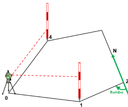
Figura 4 – Ejemplo de Rumbo 2-1 SE em la poligonal.
