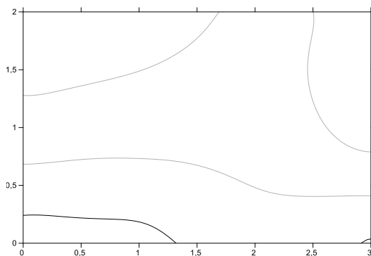
Figura 2 – Curvas de nivel dibujadas a 200 m, 300 m y 400 m, a través de los Puntos Cotizados.
