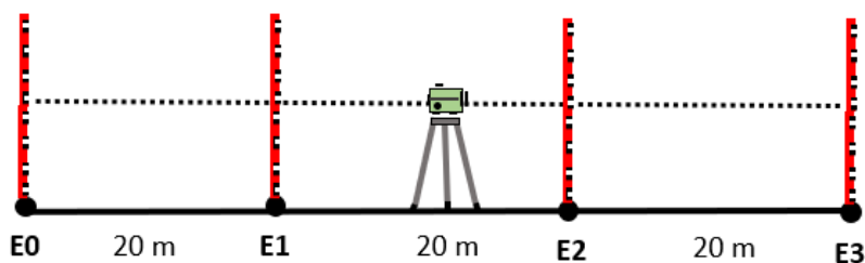
Figura 35 – Nivelamento Geométrico do Perfil Longitudinal.
