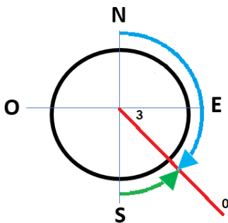
Figura 6 – Azimute e Rumo no quadrante Sudeste.
