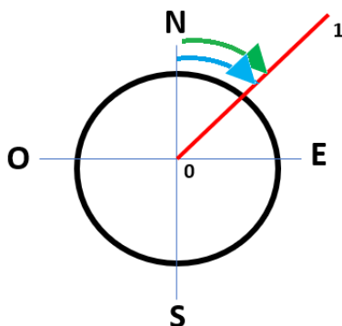
Figura 5 – Azimute e Rumo no quadrante Nordeste.
