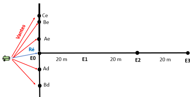
Figura 40 – Determinação das Cotas e Altitudes da Seção 0.
