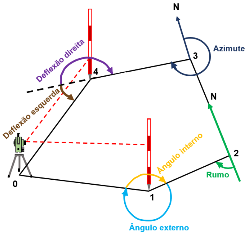
Figura 2 – Ângulos horizontais: diretos, azimute, rumo e deflexões.
